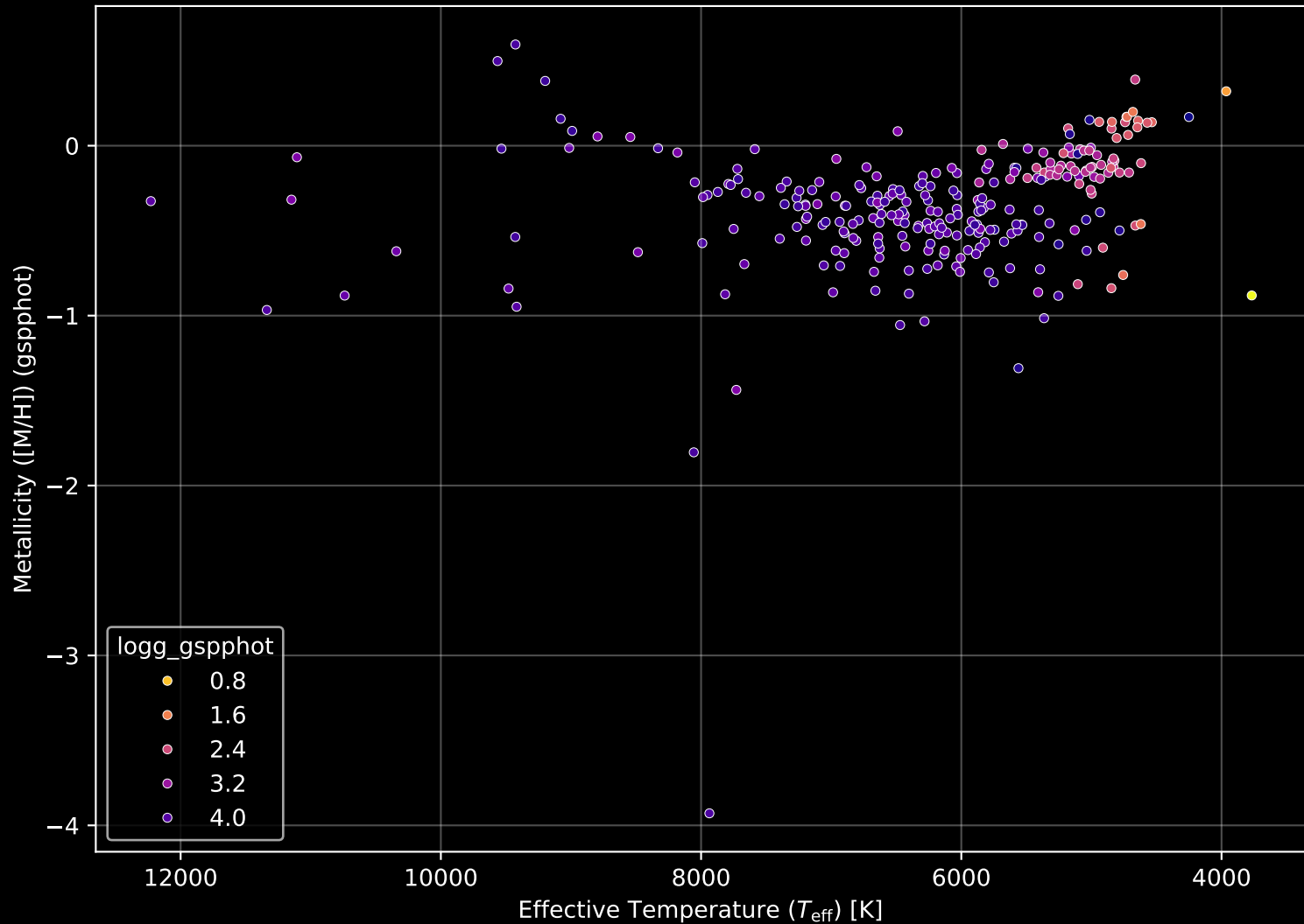
GALAH DR4 Field: [9395] Stellar Population Parameters (n= 271)
