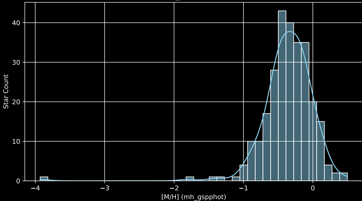
GALAH DR4 Field: [9395] [M/H] (mh_gspphot) (n= 270)
