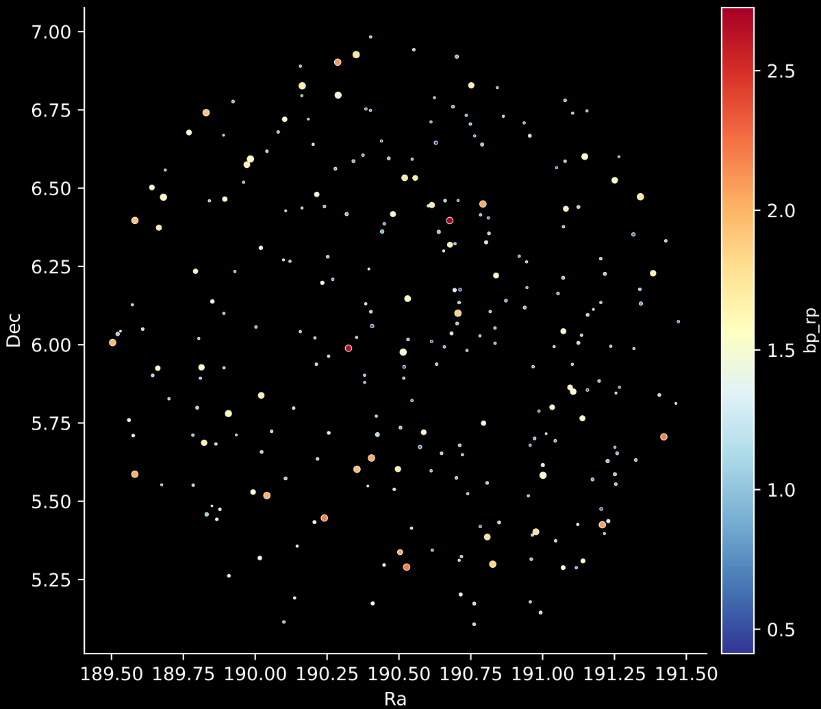
GALAH DR4 Field: [9395] Stars: 271
