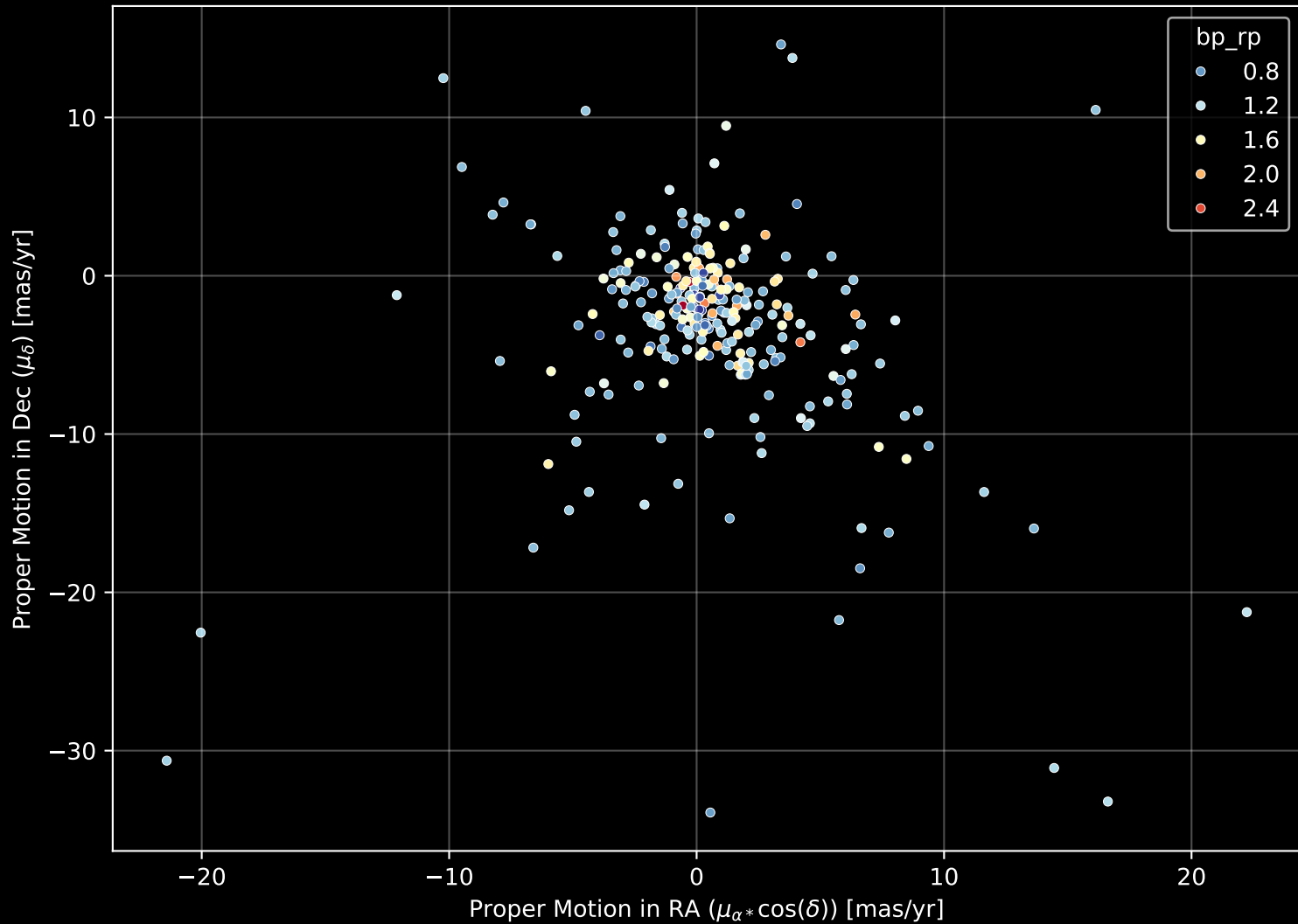
GALAH DR4 Field: [9395] Proper Motion Diagram (n= 271)
