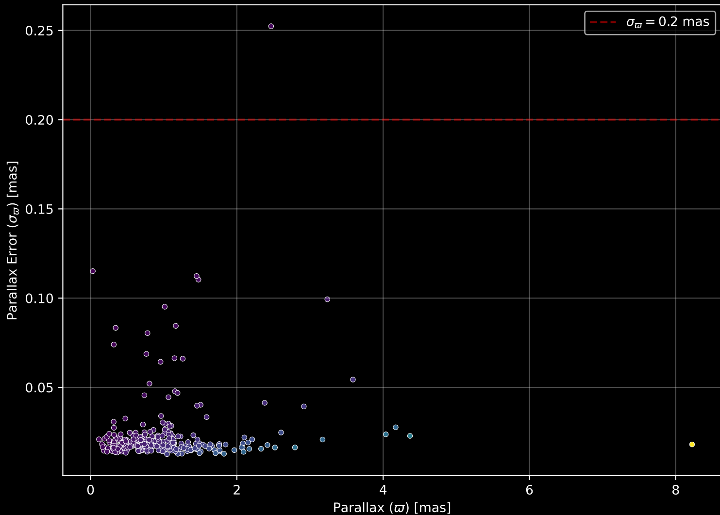
GALAH DR4 Field: [9395] Parallax Quality (n= 271)
